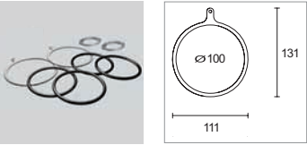
NET.SO 28 RAL 7035 Sospensione (coppia). Suspension (pair). Suspension (couple).
