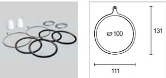
NET.SO 07 Sospensione (coppia). Suspension (pair). Suspension (couple).
