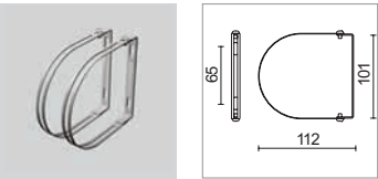
NET.AP2 Attacco a parete o plafone (coppia). Wall/ceiling mount (pair). Fixation plafond/murale (couple).
