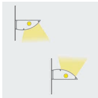
Alcune possibilità di installazione dell'apparecchio, per creare illuminazione diretta o indiretta.
